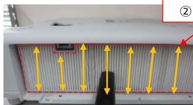
フィルタカバーを取り外した状態
